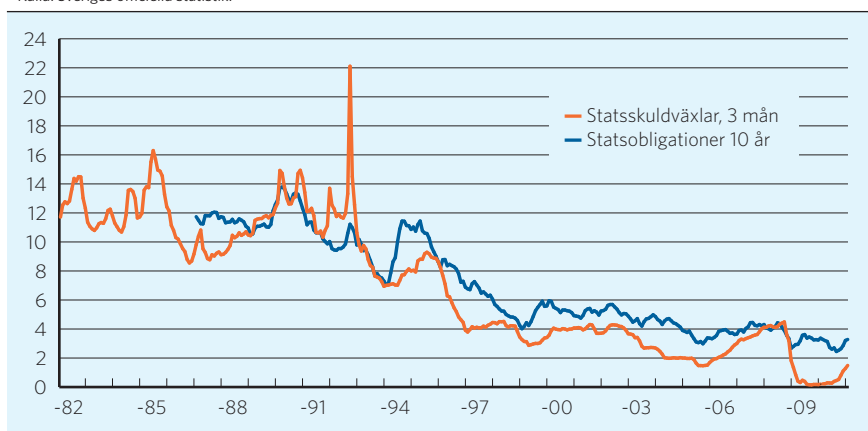
FIGUR 3: Ränteutveckling, procent.
