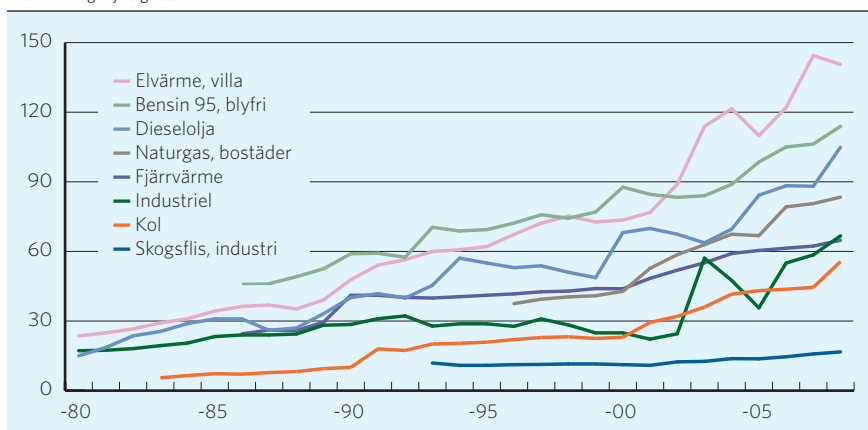
FIGUR 2: Enerprisutveckling, öre/kWh.
